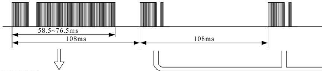
第一帧发码示意图
