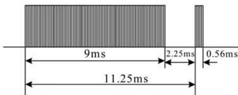
发码数据参数示意图
