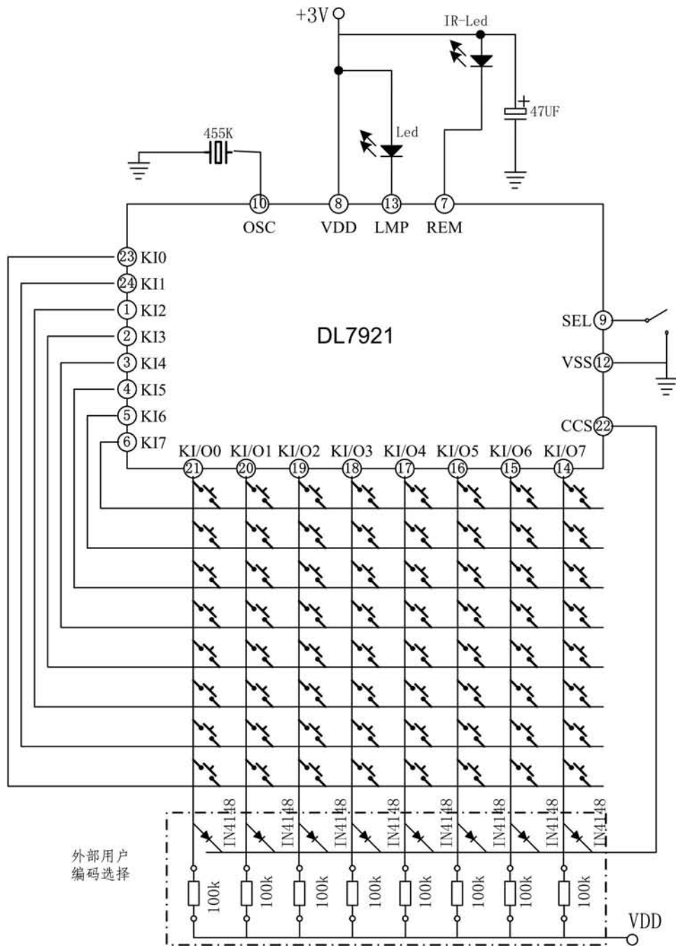
DL7921 参考应用电路图
