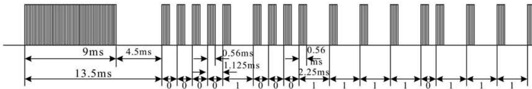
发码时间参数图
