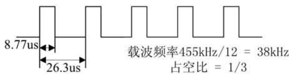
载波示意图
